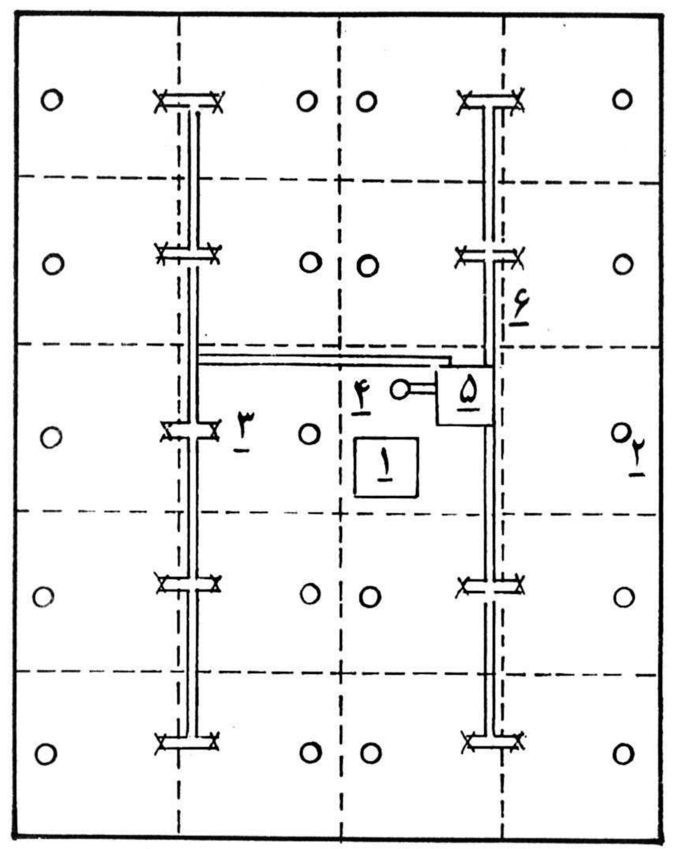
در این تصویر طریقه آبیاری با سیستم اتوماتیک مشخص شده است. در تصویر، همانگونه که می‌بینید ۶ شماره مشخص است. مخترع این سیستم آبیاری در مورد شماره‌ها چنین توضیح داده است: ۱- واحد مرکزی. ۲- واحد های خارجی (انزازه‌گیری رطوبت). ۳- شیرهای مغناطیسی آب. ۴- پمپ آبیاری. ۵- منبع آب (شوری است). ۶- لوله یابوی آب.
